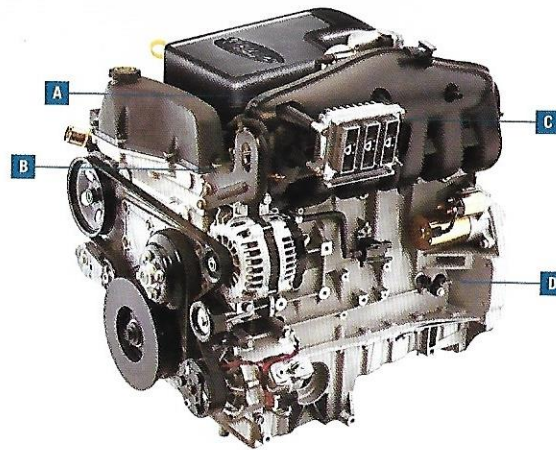
Vortec 4200 inline six
