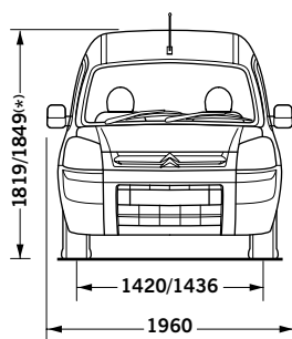
*Vehicle with Modutop®
