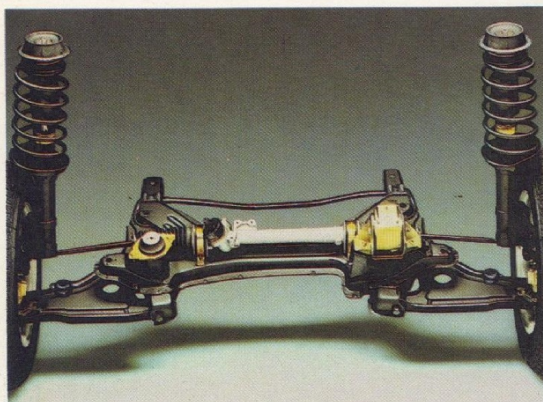
Sistema de suspensión independiente. - Provisto de barras estabilizadoras, proporciona suave marcha y estabilidad direccional.
