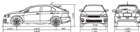
LANCER GSR SPORTBACK DIMENSIONS (MM)
