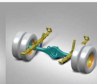
後懸吊使用葉片彈簧 + 氮氣充填減震筒
