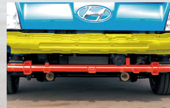
高強度底盤
