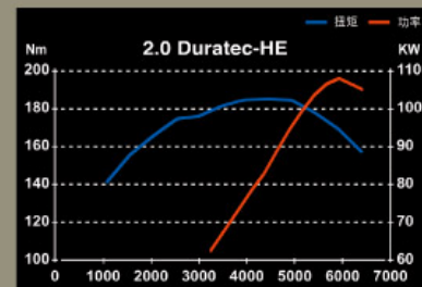
2.0L发动机性能曲线图
